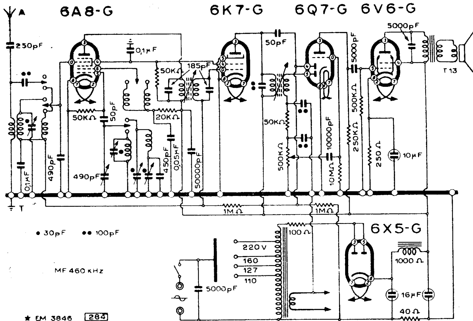
WATT RADIO - MOD. « AURORA »
